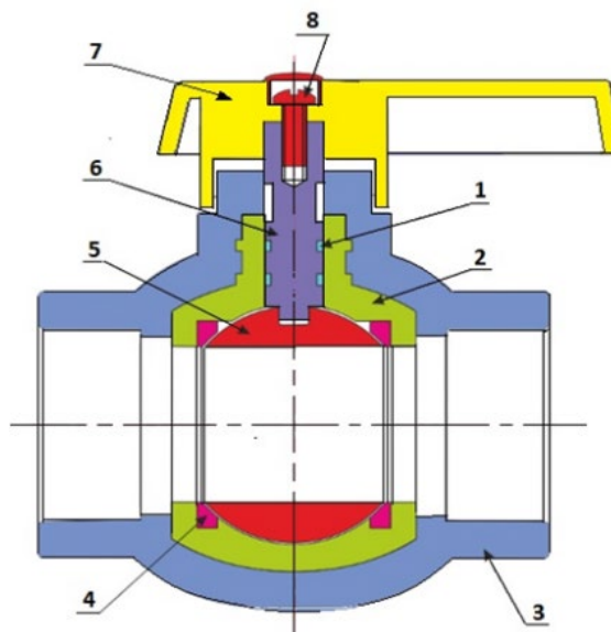
Рис.4-Конструкция шарового крана
