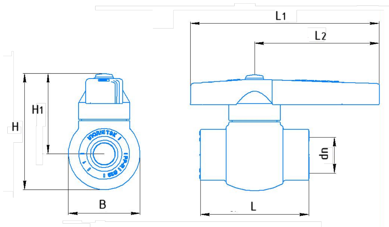
Рис 1- Кран шаровой стандартно проходной., исполнение ручка.
