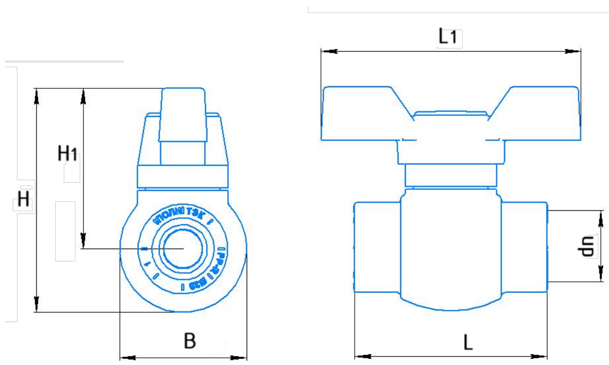
Рис 2 - Кран шаровой стандартно проходной., исполнение ручка- бабочка.
