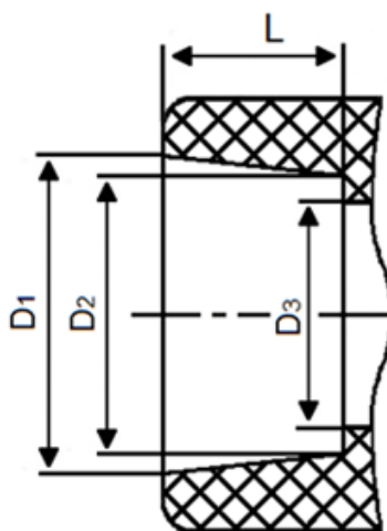
Рисунок 2- Раструбная часть корпуса шарового крана
